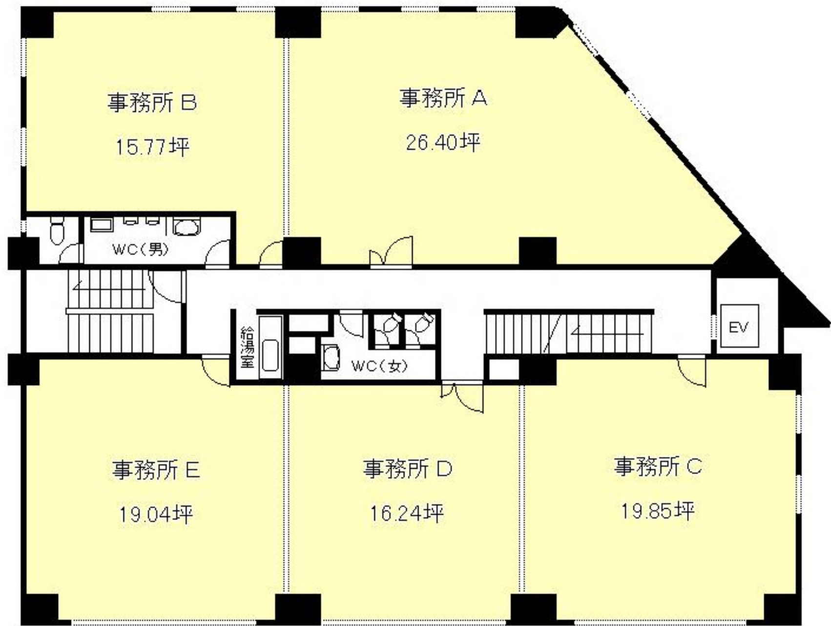
3階～7階 平面図
