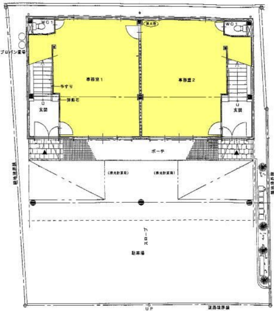
1階 平面図
